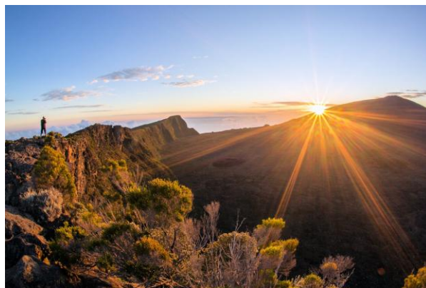
Vulkan Piton de la Fournaise
